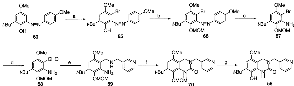
Scheme 2. (a) \text{Br}_2 , \text{CS}_2 ; (b) \text{MOMCl} , \text{NaH} , \text{DMF} ; (c) \text{H}_2 , \text{Pd-C} , \text{MeOH} ; (d) (1) n - \text{BuLi} , \text{Et}_2\text{O} , (2) \text{DMF} ; (e) (1) 3-(aminomethyl)pyridine, \text{benzene} , (2) \text{NaBH}_3\text{CN} , \text{CH}_3\text{CN} ; (f) triphosgene, \text{Et}_3\text{N} , \text{CH}_2\text{Cl}_2 ; (g) \text{conc'd HCl} , \text{MeOH} .
